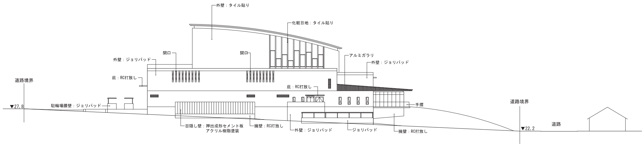
南側立面図
