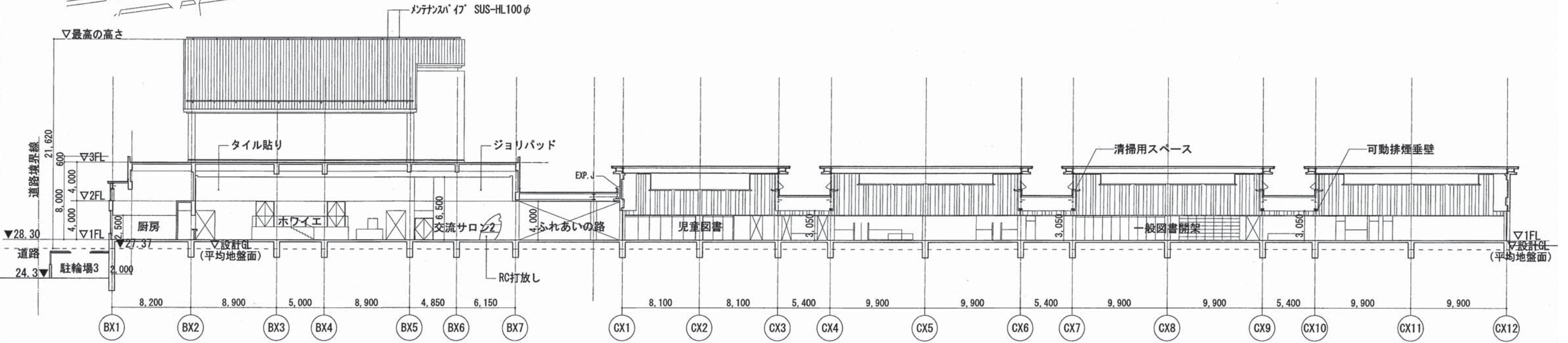
C-C断面図
