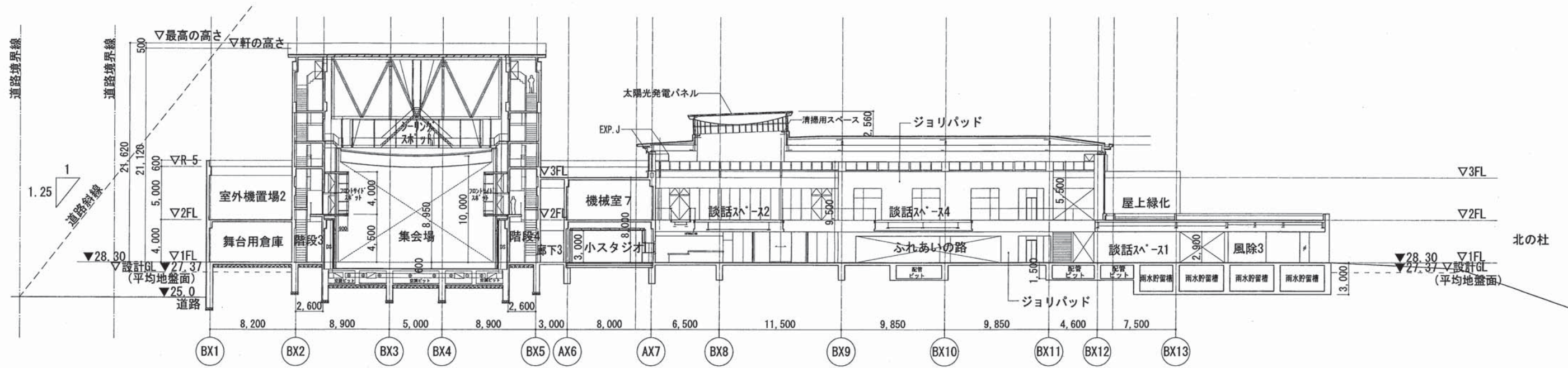
D-D断面図
