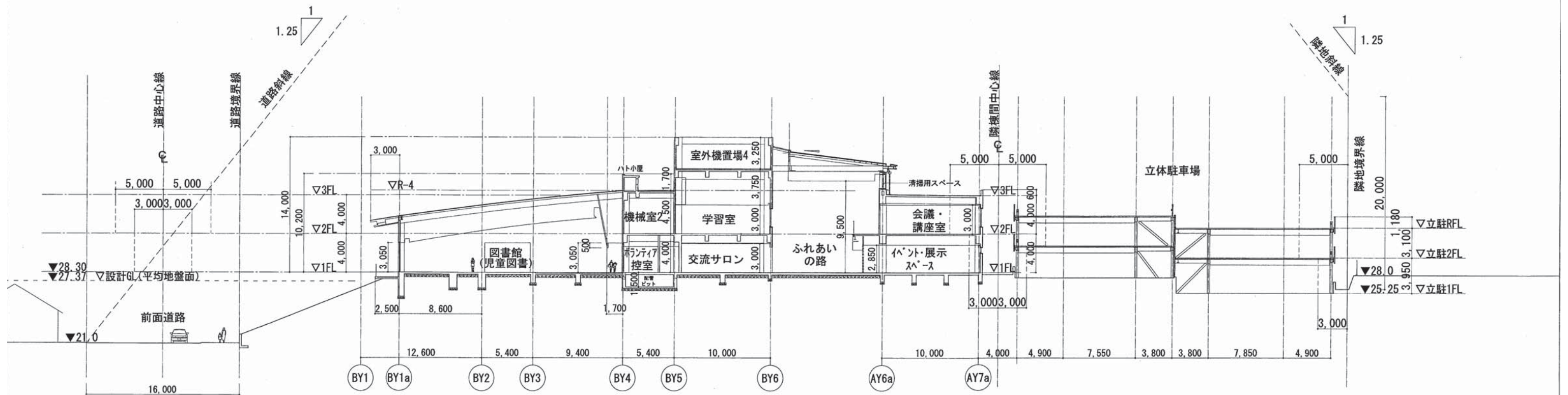
B-B断面図
