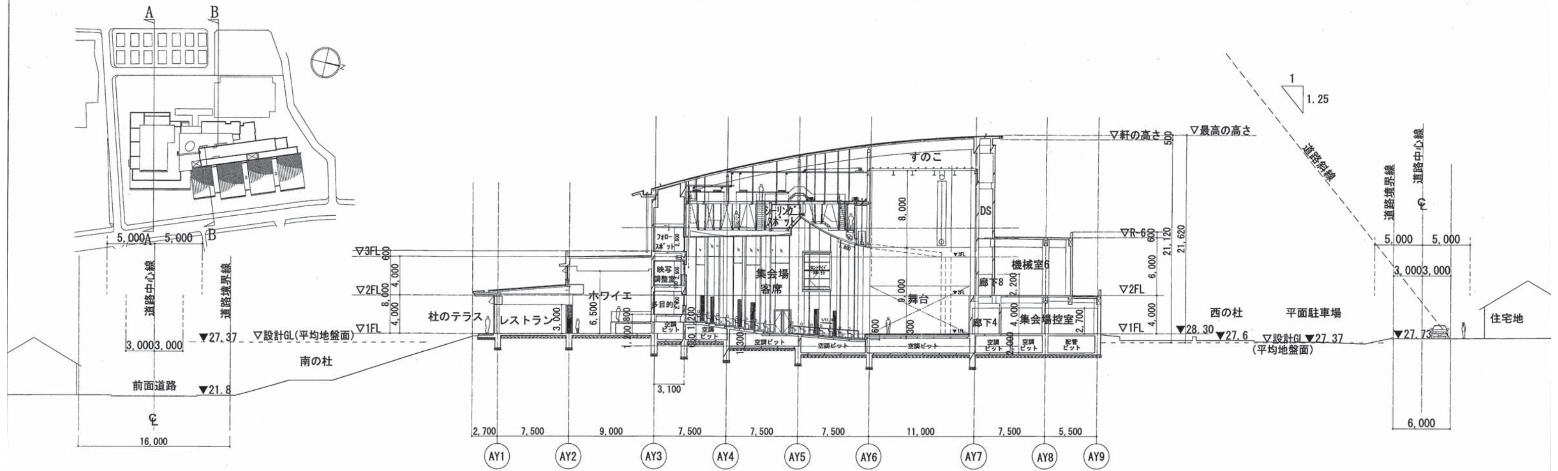
A-A断面図
