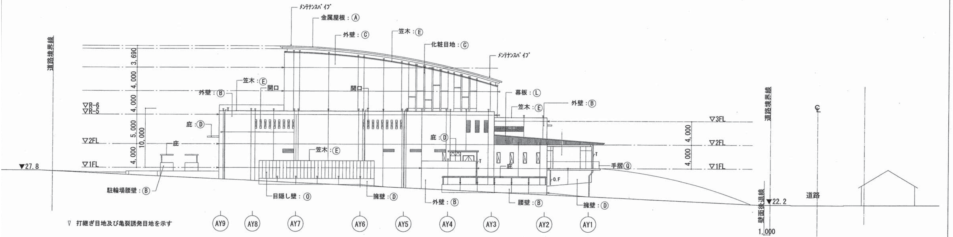
南側立面図
