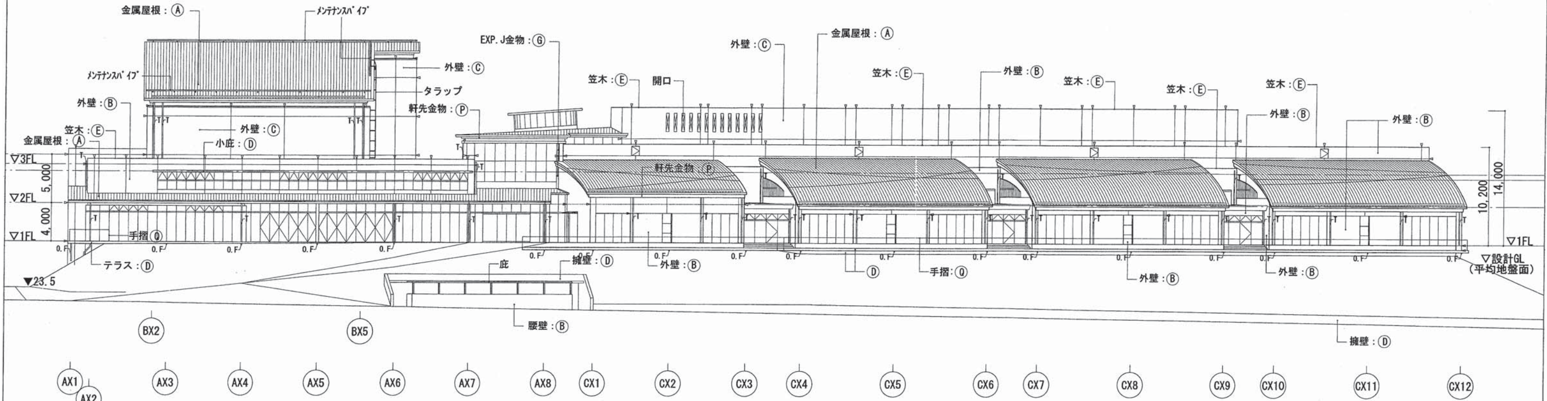
東側立面図
