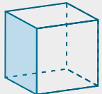
▲立方体
