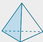
▲正四面体
