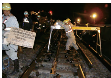
【レール更换】レールを新しく更换する作業
