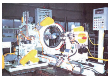
造機写真
